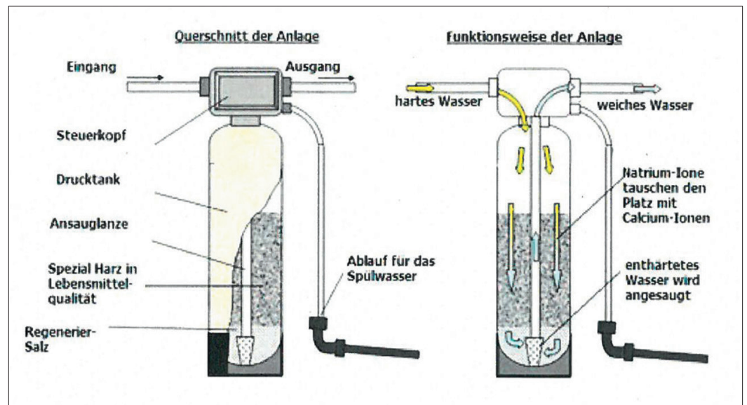
Funktionsweise einer Wasserenthärtungsanlage mittels Ionenaustausch.
